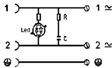
bipolare LED und RC Schutzbeschriftung
