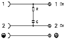
RC-Schutzbeschriftung
