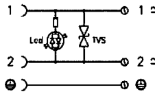
bipolare LED und Schutzbeschriftung Transil-Diode
