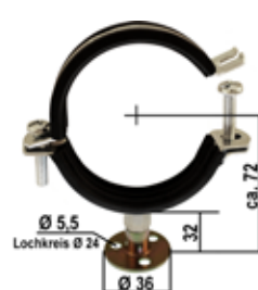
Für Größe 11/2"
