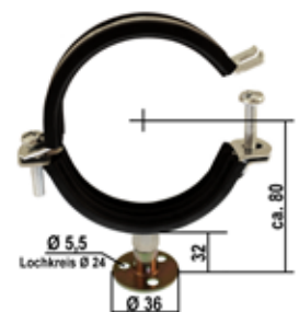
Für Größe 2"
