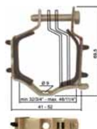
Für Größe 3/4"-11/4"
